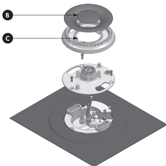
B - Brûleur coupe C - Épandeur Gaz Brûleurs
