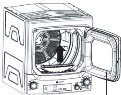
Filtre à charpie derrière la grille
