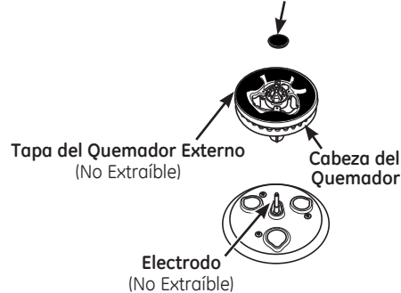
Tapa del Quemador Interno (Extraíble)
