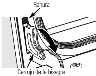
Jale hacia abajo los cerrojos de la bisagra para desbloquear
