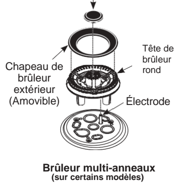
Chapeau de brûleur interne (Amovible)
