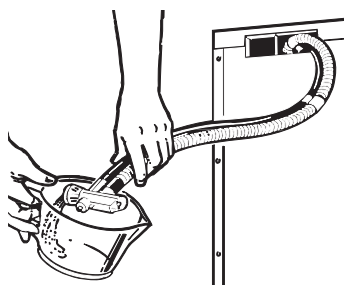
Appuyez sur le collier pour débrancher le raccord unicouple du robinet
