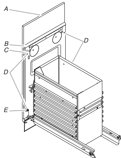
A. Panneau personnalisé B. Quart-de-rond de 15" x \frac{1}{2} " C. Façade du tiroir D. Position des quatre vis à bois n° 8 x 1" E. Butée de caoutchouc (une de chaque côté)
