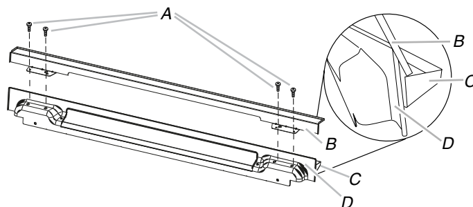
A. Vis n° 8-18 x 1/4" B. Support du déflecteur
