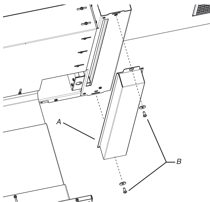
A. Plateau d'égouttement B. Vis (2)
