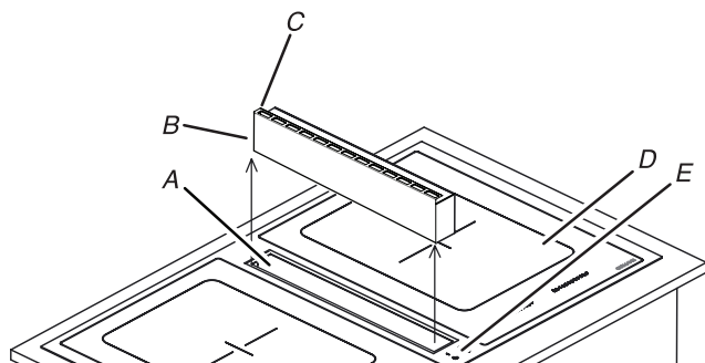
A. Porte du système d'extraction B. Filtre du système d'extraction C. Poignée du filtre D. Table de cuisson E. Commandes du système d'extraction
