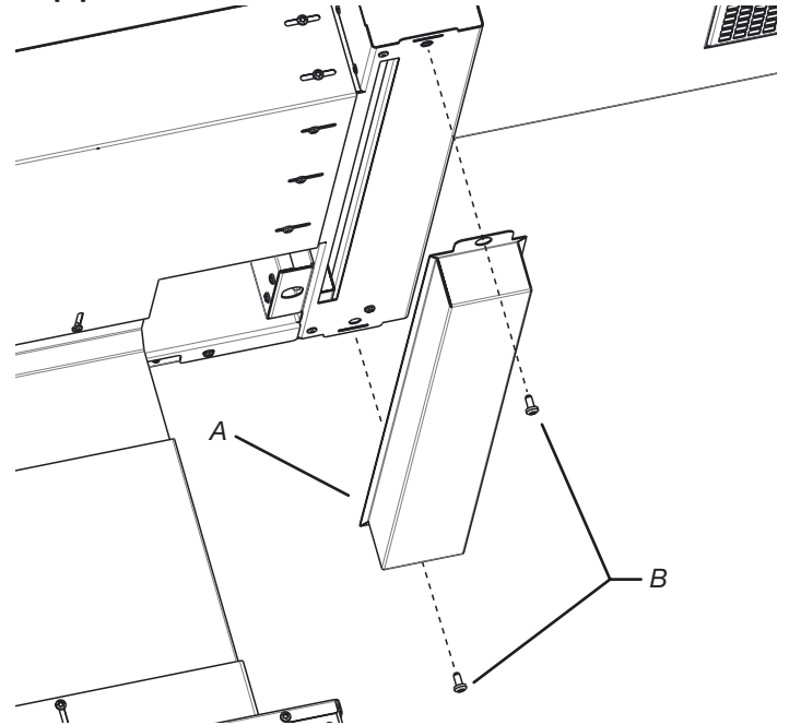
A. Drip pan B. Screws (2)
