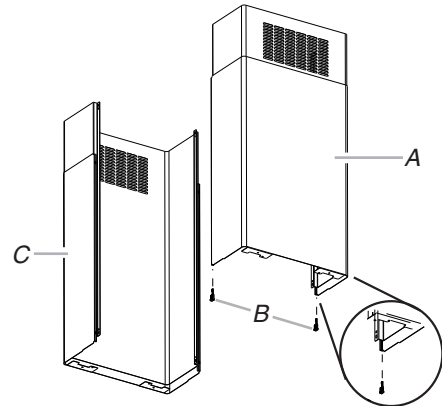
A. Assemblage de la partie supérieure et de la partie inférieure du cache-conduit - (placement à l'avant) B. Chevilles en plastique (2) (extrémité longue pour placement à l'avant) C. Assemblage de la partie supérieure et de la partie inférieure des cache-conduits - (placement à l'arrière)
