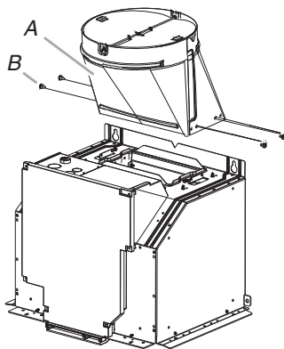
A. Raccord de transition B. Vis de 4 x 8 mm
