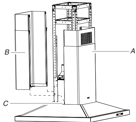
A. Cache-conduit (assemblage avant) B. Cache-conduit (assemblage arrière) C. Chevilles en plastique (2) à l'avant de la partie inférieure du cache-conduit
