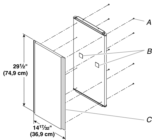
A. Tornillo para madera de cabeza de cono achatado #8 x \frac{1}{2} " B. Almohadillas adhesivas C. Panel hecho a la medida
