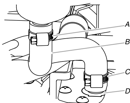
A. Abrazadera ajustable para manguera, de \frac{5}{8} "
