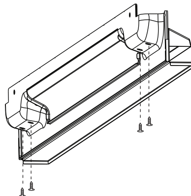
Assemblage de l'évent du four depuis la partie inférieure arrière
