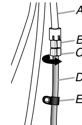
A. Línea de agua de plástico B. Puerto de entrada de la válvula de agua C. Tuerca de compresión D. Tubería de cobre E. Abrazadera en "P"
