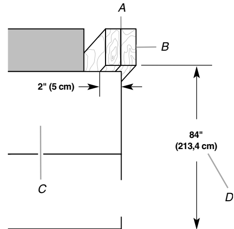
A. Deux planches de 2" x 4" x 32" (5 cm x 10 cm x 81 cm)
