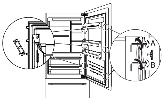
A. Réglage de la vis à épaulement B. Réglage de la vis de blocage
