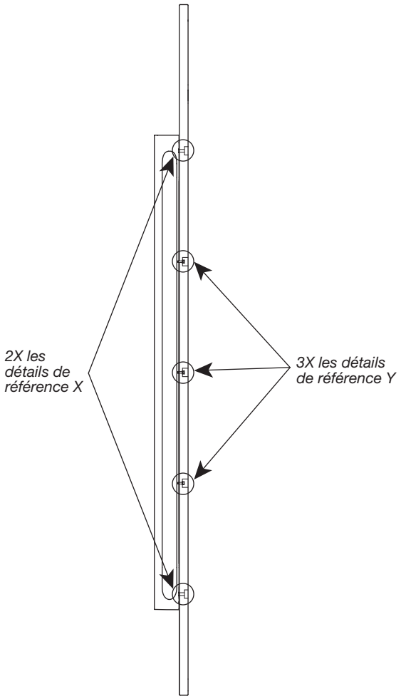
Illustration 2 - Vue transversale
