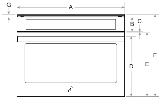
VUE AVANT
