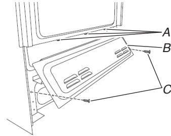
A. 3 onglets de montage B. Couvercle d'accès inférieur C. (2) vis
