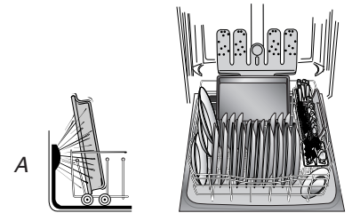
A. Parte posterior de la lavavajillas
