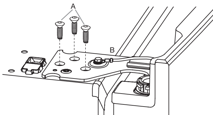
A. Tornillos TORX® T25®
