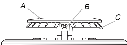
A. Burner cap B. Electrode C. Burner base
