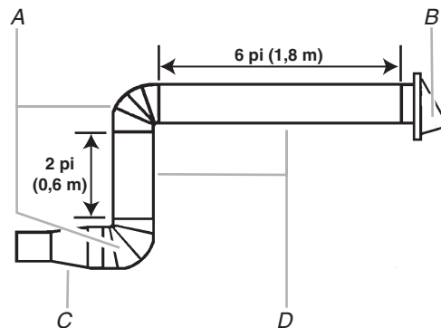
A. Deux coudes à 90° = 20 pi (6,1 m)
