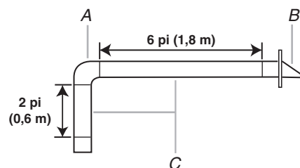
A. Un coude à 90° de 3/4" x 10" (8,3 x 25,4 cm) = 25 pi (7,6 m)
