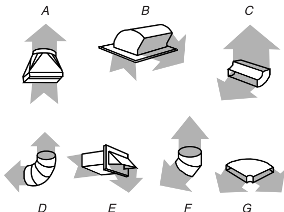
A. Raccord de transition rectangulaire/rond : 3/4" x 10" à 6" = 5 pi (8,3 x 25,4 cm à 15,2 cm = 1,5 m)
