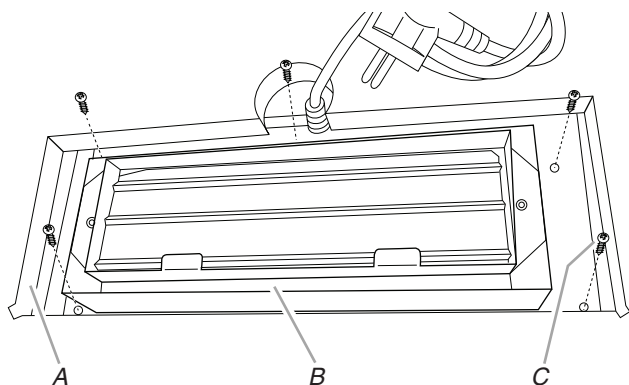
A. Clapet anti-retour B. Ouverture découpée dans le placard supérieur C. Vis métalliques de 9,5 mm (5)
