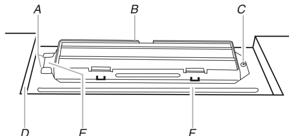
A. Pattes d'arrimage relevées B. Module du clapet anti-reflu C. Vis à tôle de 6 x 3/8" D. Ouverture découpée dans le placard supérieur E. Patte longue F. Plaque de support du clapet
