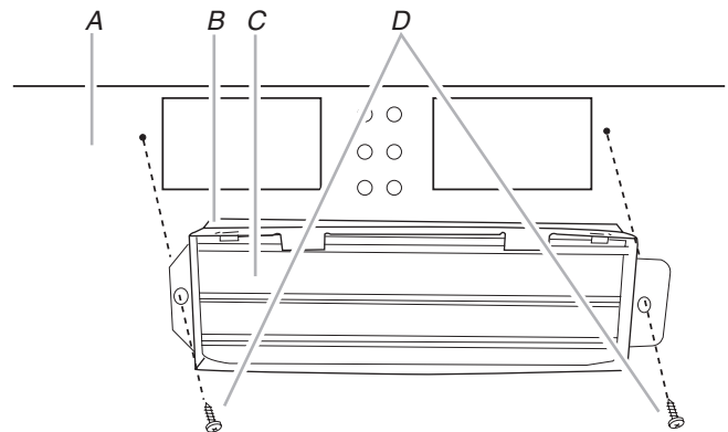
A. Face arrière du four à micro-ondes B. Module du clapet anti-reflu C. Lame du clapet anti-reflu D. Vis à tête de 6 x 3/8" (2)
