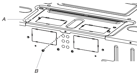
A. Plaque de support du clapet B. Introduire
