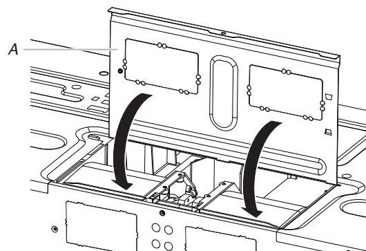
A. Plaque de support du clapet
