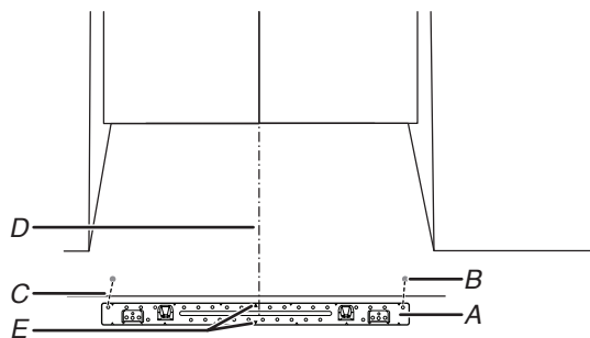
A. Plaque de montage B. Trous A et B C. Ligne du bas de la plaque de montage D. Marque centrale E. Marquage du centre sur plaque de montage
