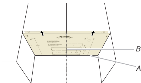
A. Bord arrière de la plaque de carton et bord arrière de l'armoire supérieure B. Axe central de l'armoire supérieure et marques centrales sur la plaque de carton
