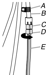
A. Abrazadera en "P" B. Línea de agua de plástico C. Puerto de entrada de la válvula de agua D. Tuerca de compresión E. Tubería de cobre
