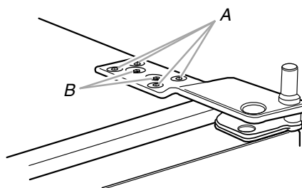
A. Tornillos de montaje de cabeza plana Torx® 27 B. Tornillos de montaje de cabeza hexagonal de \frac{1}{4} "
