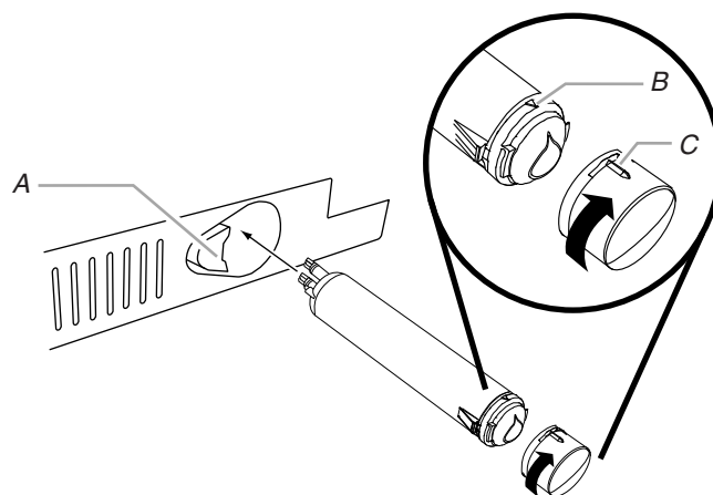
A. Bouton d'éjection
