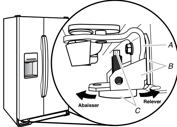
A. Charnière inférieure B. Support de vérin C. Pied de nivellement
