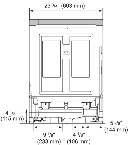
VUE ARRIÈRE
