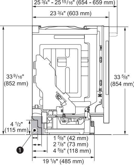
VUE AVANT
