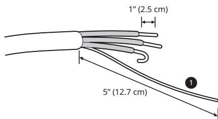
1 Fil de masse
