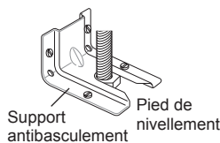
Support antibasculement Plaque murale La vis doit pénétrer dans le bois ou le béton.
