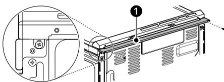
① Élément de remplissage arrière
