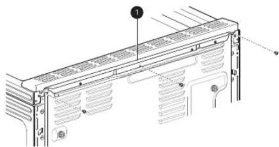
❶ Plaque arrière supérieure
