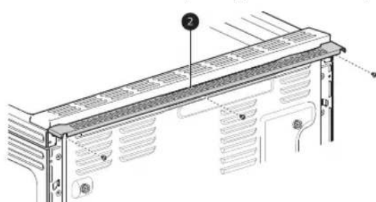
❷ Élément de remplissage arrière
