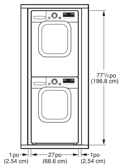
Dimensions requises pour installation avec trousse d'empilage
