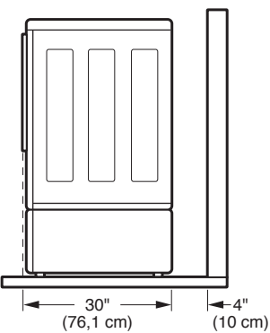
Dimensiones requeridas para la instalación con pedestal
