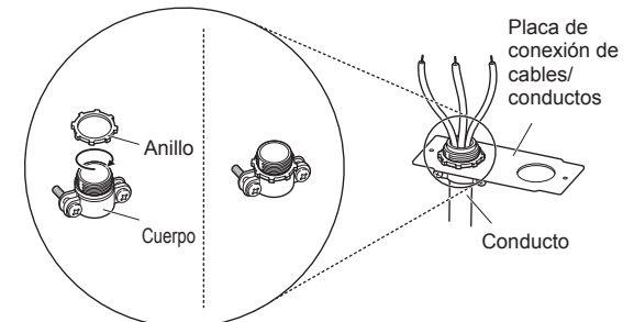
Montaje del pasacables del conducto en la abertura de 1 1/8"
