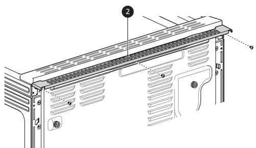
2 Placa trasera
