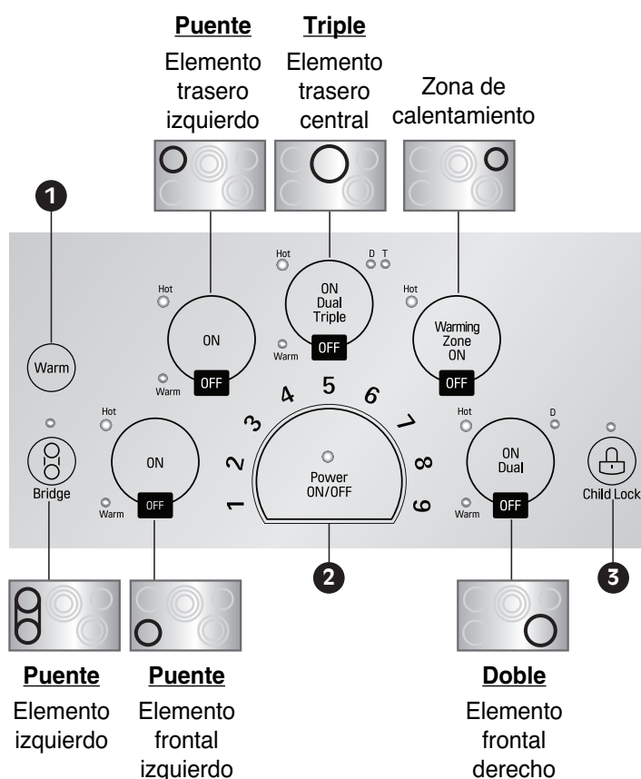
Estufa radiante UPCE3664ST
