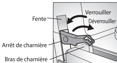
Arrêt de charnière ouvert
