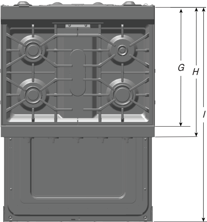
VISTA SUPERIOR
