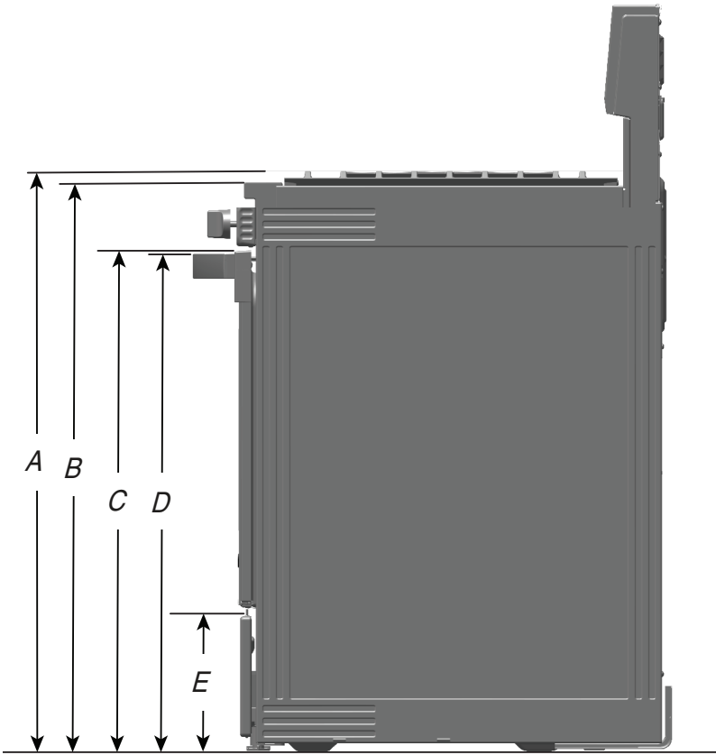
VISTA LATERAL
