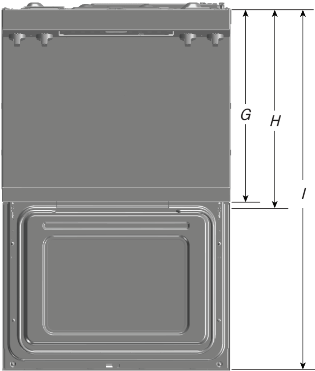
VISTA SUPERIOR
