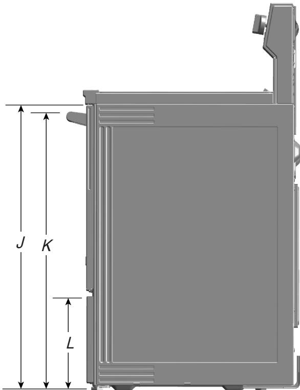
VISTA LATERAL
