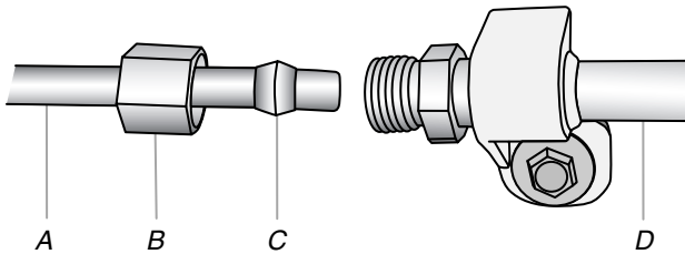
A. Línea de agua de la casa C. Férula (adquirida) B. Tuerca (adquirida) D. Tubería de agua del refrigerador
