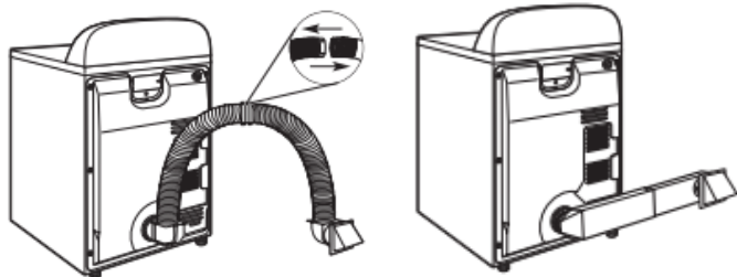
Installation au-dessus de la sècheuse Installation en périscopie (également offerte avec un coude décalé)
