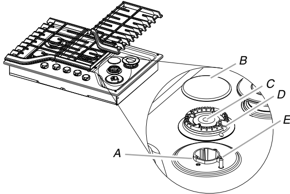
A. Porte-gicleur B. Chapeau du brûleur C. Ouverture du tube de gaz D. Base du brûleur E. Electrode d'allumage
