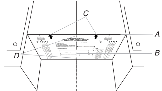
A. Bord avant du gabarit de l'armoire supérieure et bord avant de l'armoire supérieure B. Axe central de l'armoire supérieure C. Flèches sur le gabarit de l'armoire supérieure D. Centrer les repères sur le gabarit du haut de l'armoire
