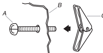
A. Perno de cabeza redonda de 3/16-24 x 3" B. Placa de montaje C. Tuerca de palanca con resorte
