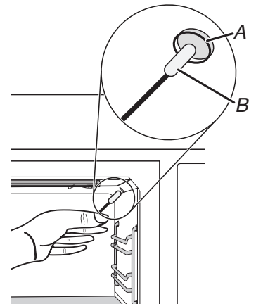
A. Lentille du capteur infrarouge B. écouvillon non pelucheux avec lentille
