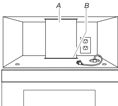
A. Système d'extraction B. Clapet antiretour (sous le conduit d'évacuation)
