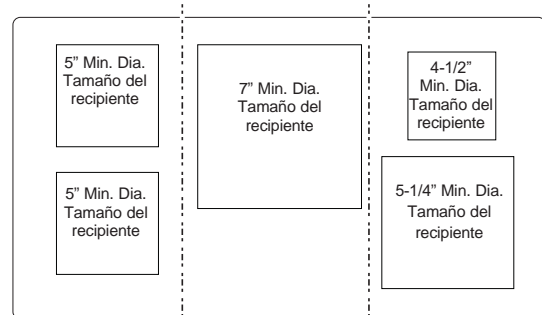
Placa de cocción de 36"
