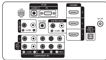
DETALLE DEL PANEL DE TOMAS 3.7"H X 9.1"W
