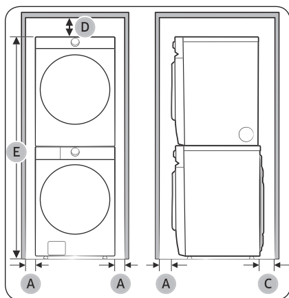
Installation superposée (Modèle : SKK-9MC*)
