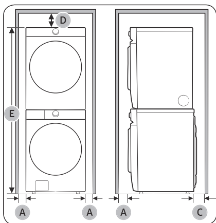
Instalación apilada (Modelo: SKK-9MC*)
