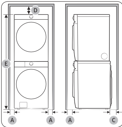
Instalación apilada
