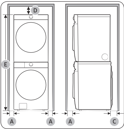
Installation superposée
